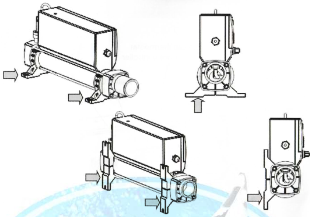
OBRÁZEK 2 Podlahová montáž – nastavení
